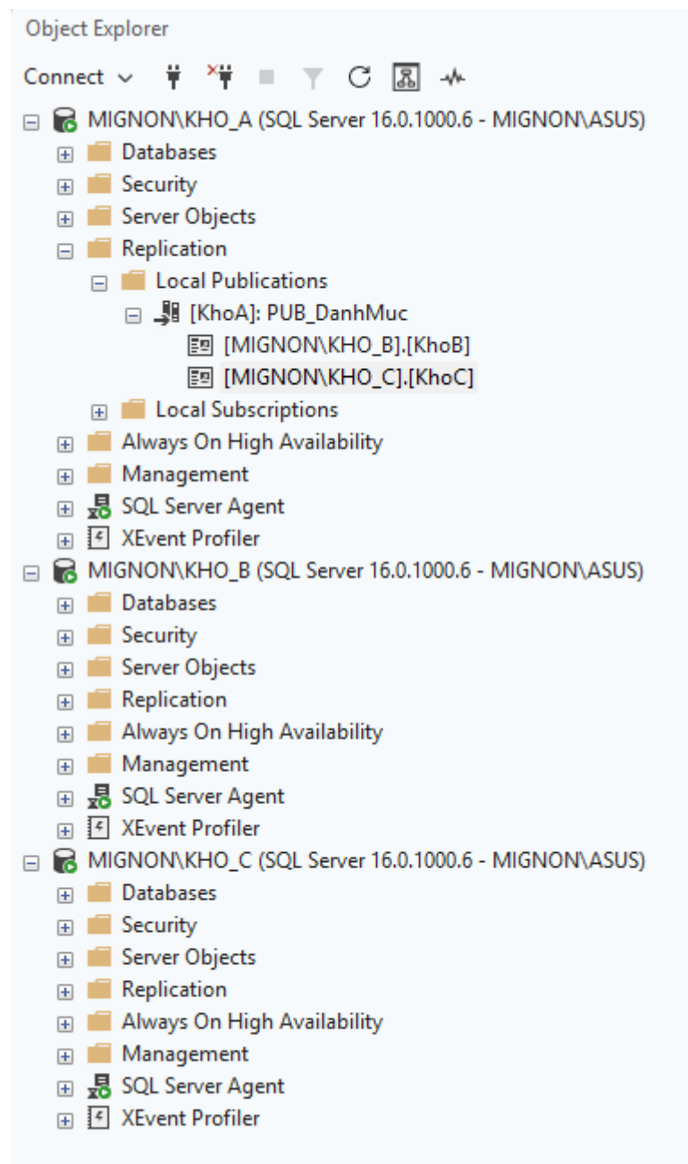
Hình 26: Publication PUB_DanhMuc trong Object Explorer tại site KHO_A
