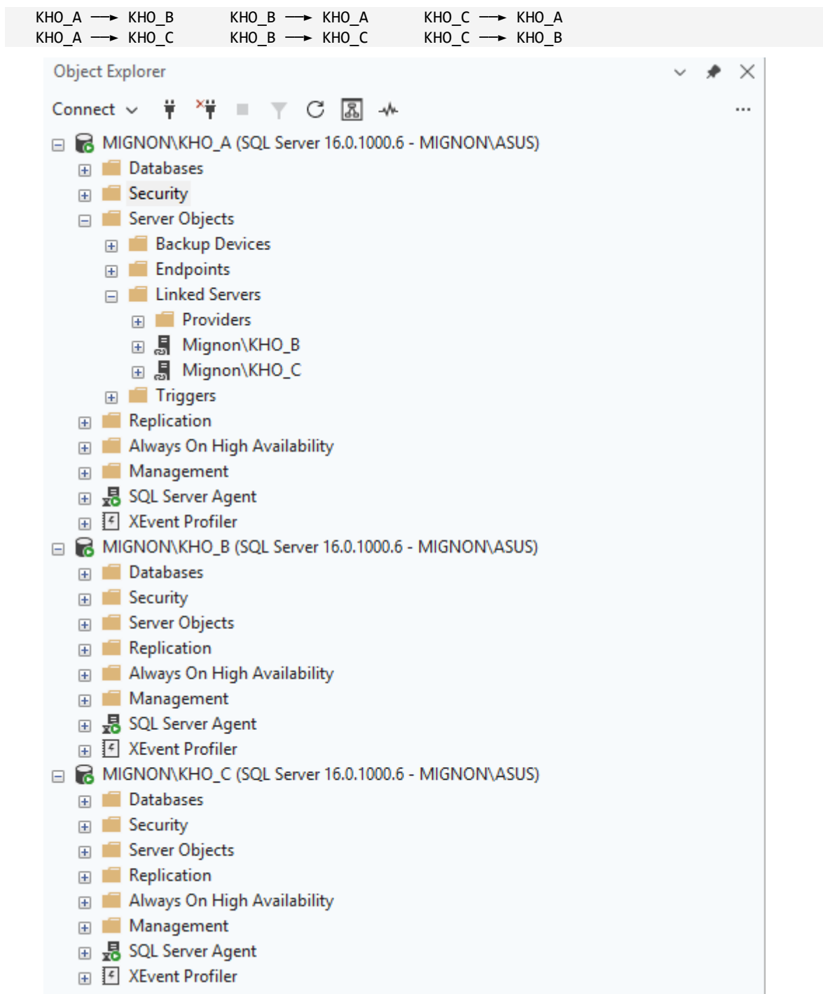
Hình 22: Hai Linked Server tại site KHO_A trong Object Explorer
